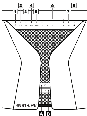
Routeur
